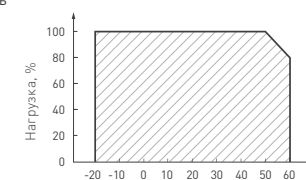
Температура окружающей среды (Ta), °C Рис. 3. Максимальная допустимая нагрузка, % от мощности источника
