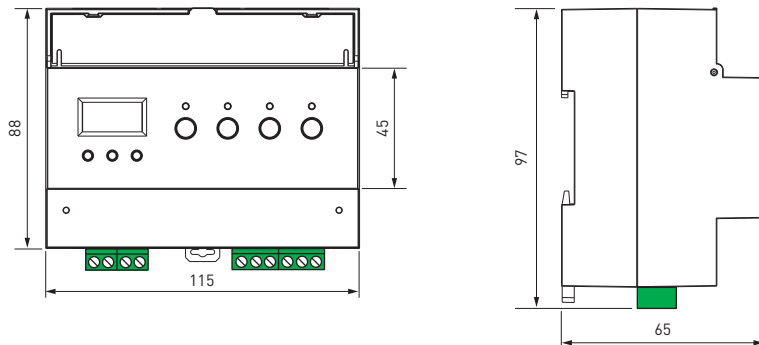
Рис. 1. Габаритный чертеж
