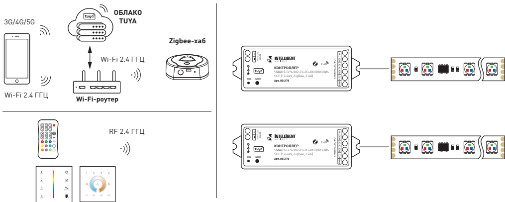
Рис. 2. Общая структурная схема построения системы управления
