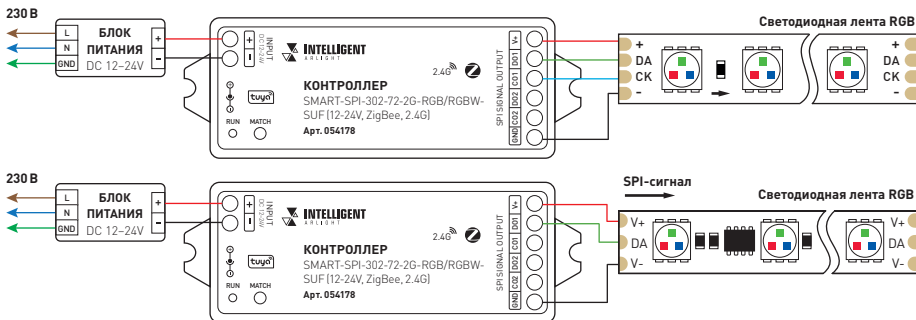
Рис. 4. Схема подключения контроллера SMART-SPI для управления светодиодной лентой SPI
