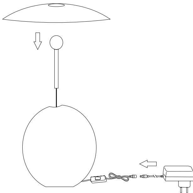
Рис. 2. Сборка светильника
